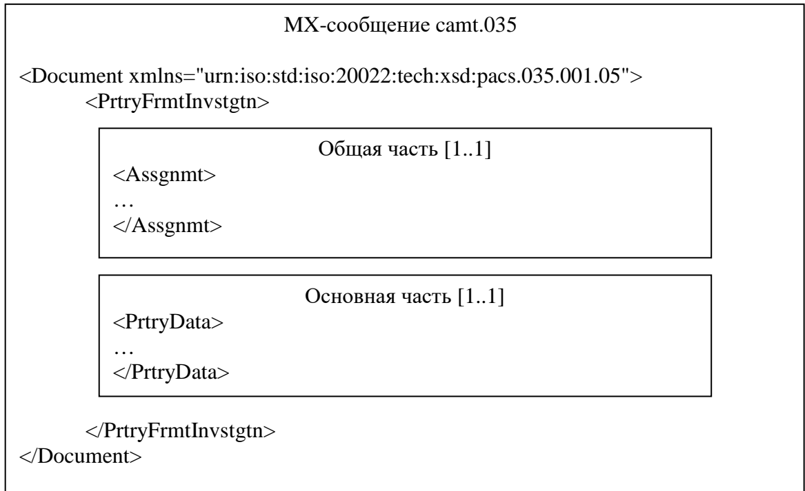
Рисунок 1 – Структура МХ-сообщения samt.035
